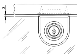
Felülre szerelt zár egyszárnyú ajtóra
