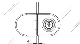
Középre szerelt 201 zár kétszárnyú ajtóra 0917.010 ellendarabbal*
