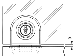
Alulra szerelt zár egyszárnyú ajtóra
