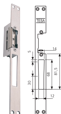
LBI Kicsapódó, ferde nyelvé zárhoz
