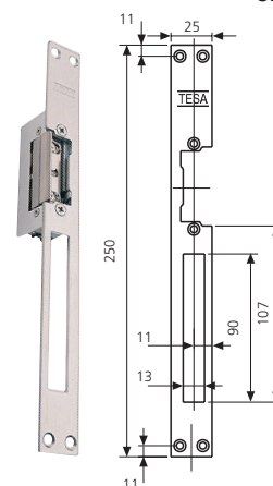
LCI Hagymányos zárnyelvű zárhoz
